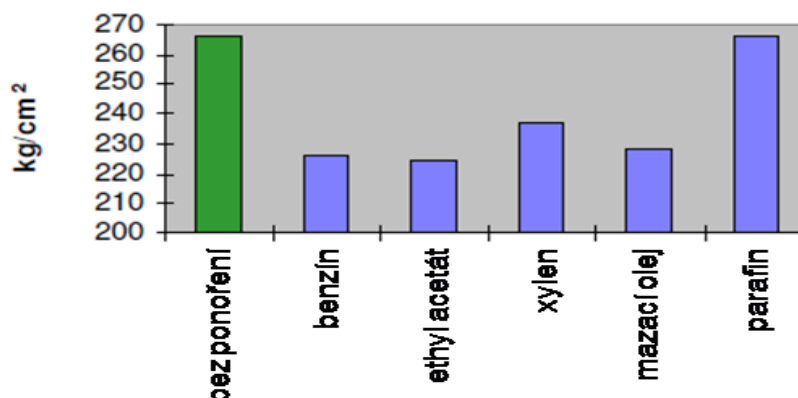
Síla přilnavosti ponořeného přípravku EPOXICEYS standard
