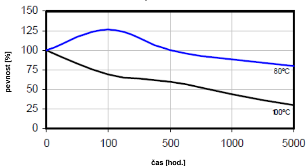
Teplené stárnutí
